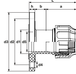
TİP-B / TYPE B
